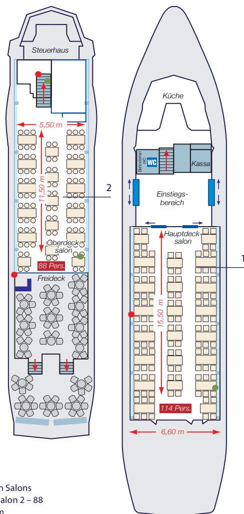
Hauptdeck
